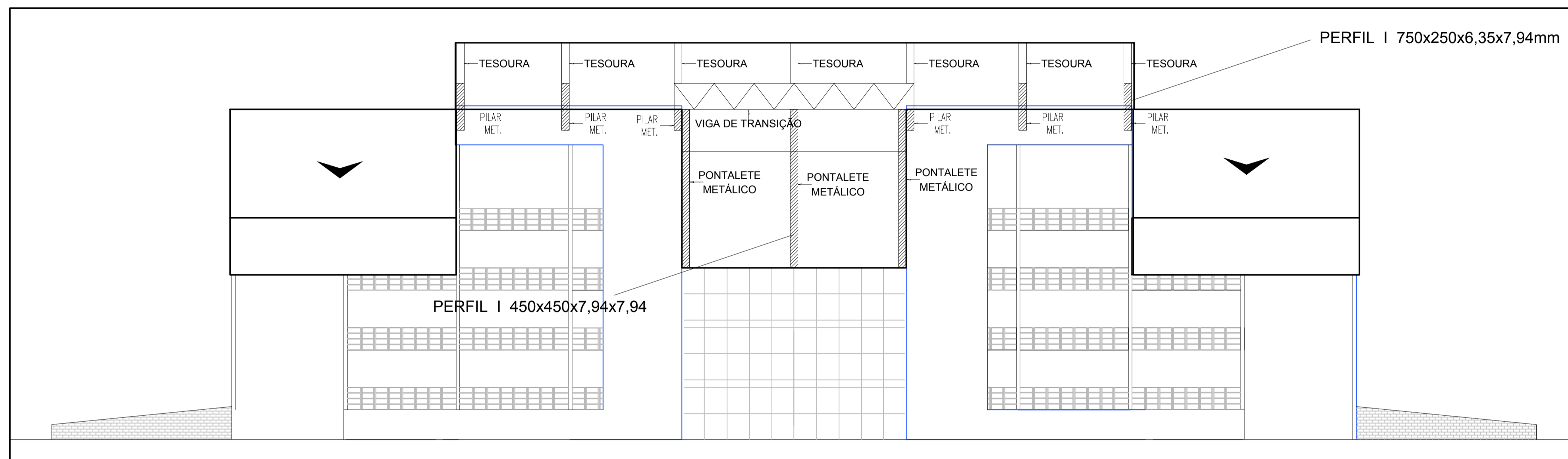
Fachada Leste - Rua do Nascente
