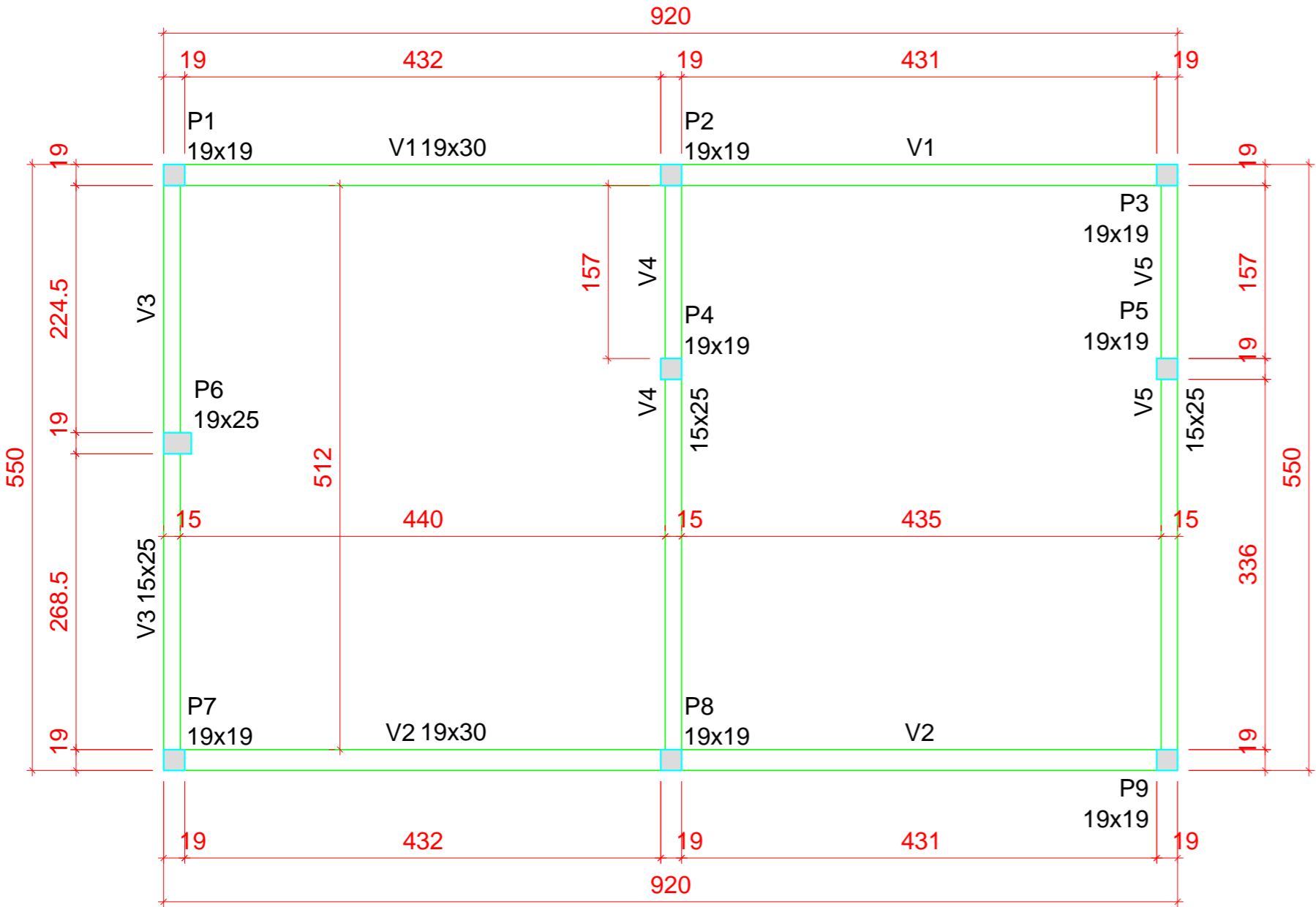
Forma do pavimento terreo (Nível 290) escala 1:50
