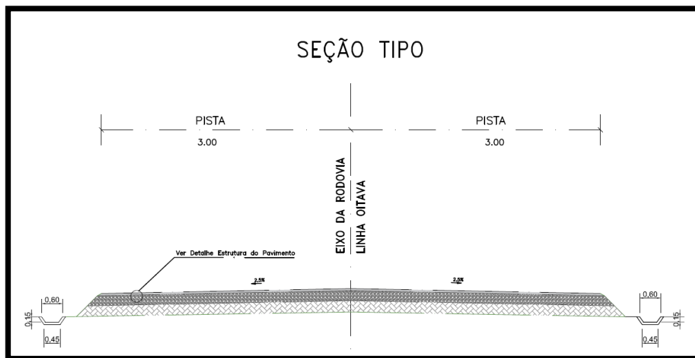
Imagem 01: Detalhamento Sarjetas Trapezoidais de concreto
