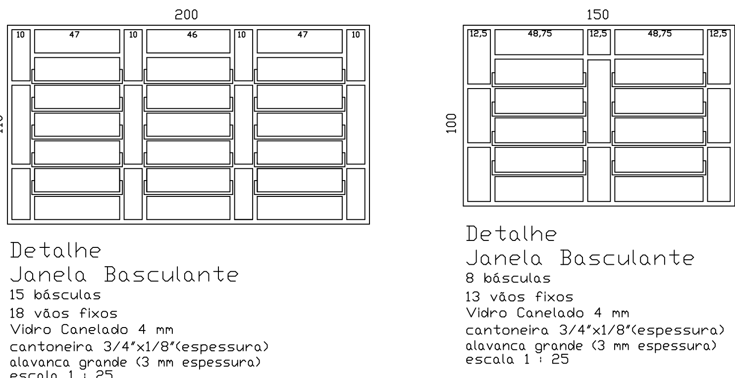
JANELAS BASCULANTES
