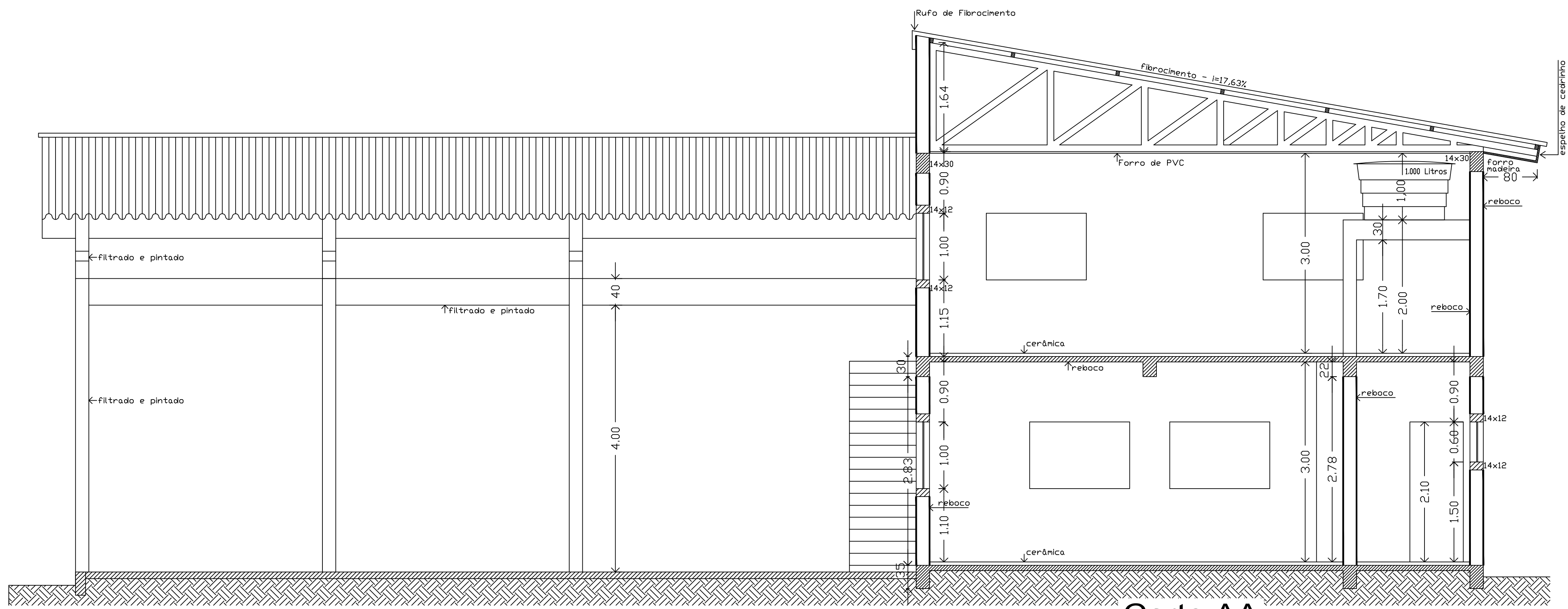
Corte AA
