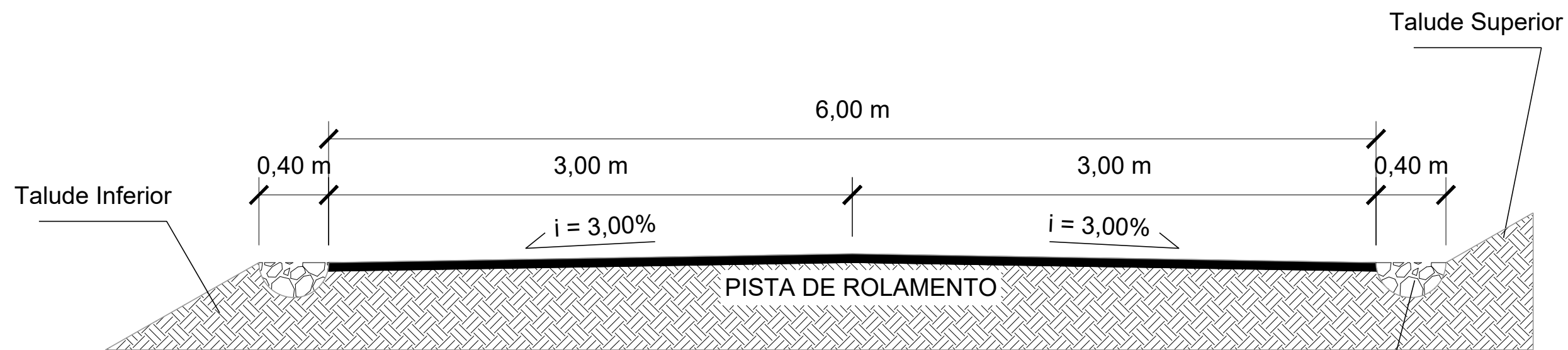
SEÇÃO TRANSVERSAL PROPOSTA
